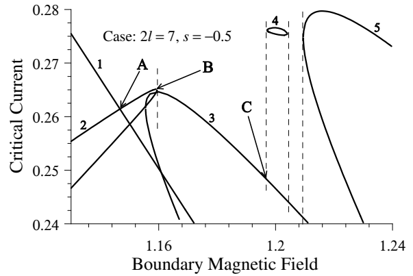
Рис. 2: Нарушения непрерывности парциальной КК для 2l = 7 и s = -0.2
