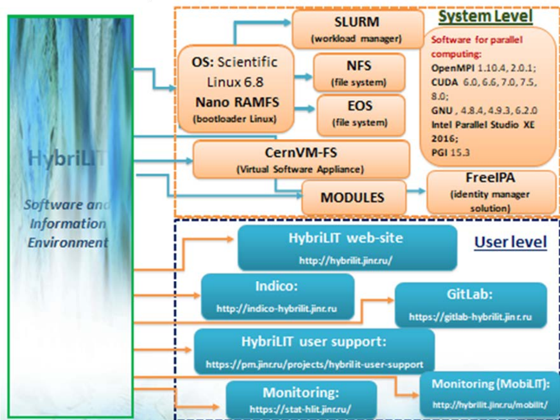
Рис.1. Программно-аппаратная среда кластера HybriLIT
