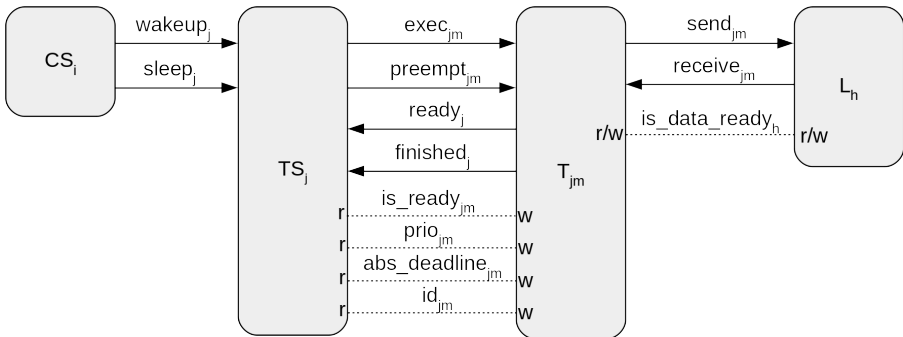
Рис. 1 — Средства взаимодействия, определенные для базовых типов автоматов в обобщенной модели функционирования МВС
